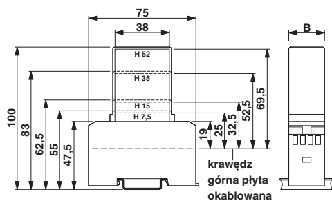
Rysunek wymiarowy
