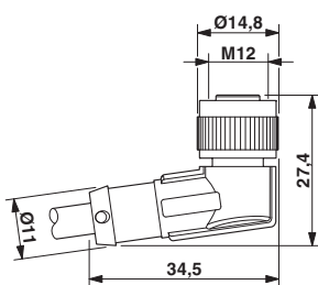
Rysunek wymiarowy
