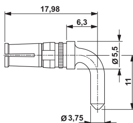
Rysunek wymiarowy
