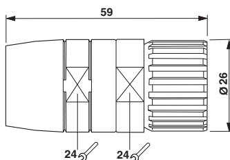
Rysunek wymiarowy
