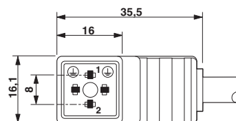
Rysunek wymiarowy
