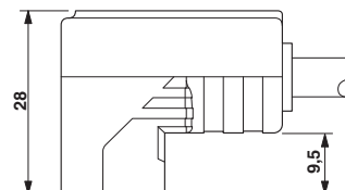
wtyk zaworowy, konstrukcja C, z boku
