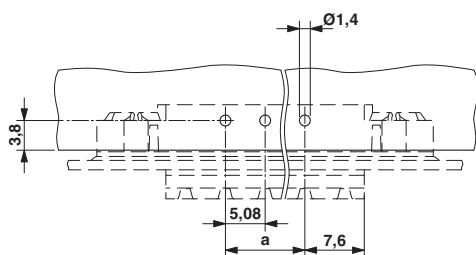
Szablon wierceń
