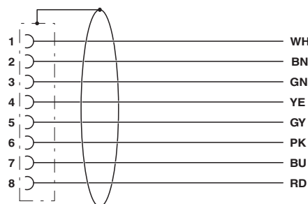
Przyporządkowanie styków gniazda M8
