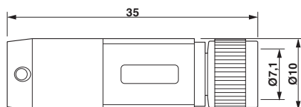
Gniazdo M8 x 1, proste
