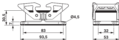
Rysunek wymiarowy
