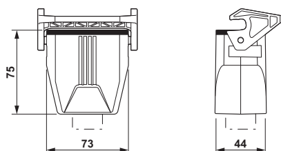
Rysunek wymiarowy
