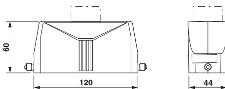
Rysunek wymiarowy
