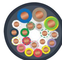
Przekrój kabla
