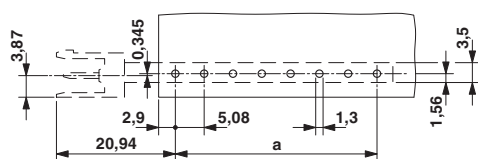
Szablon wierceń
