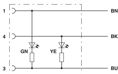
Przyporządkowanie styków gniazda M8
