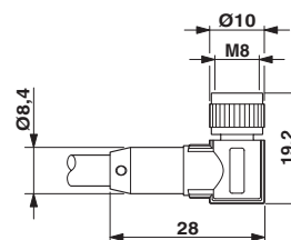
Gniazdo M8x1, kątowe, z LED
