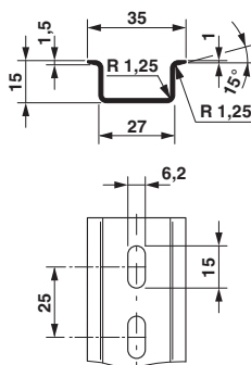
Rysunek wymiarowy
