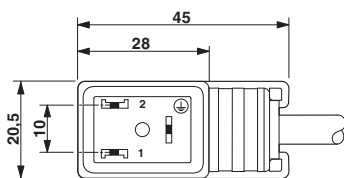
Wtyk zaworowy, typ B
