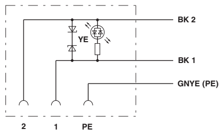
Przyporządkowanie styków wtyku zaworowego
