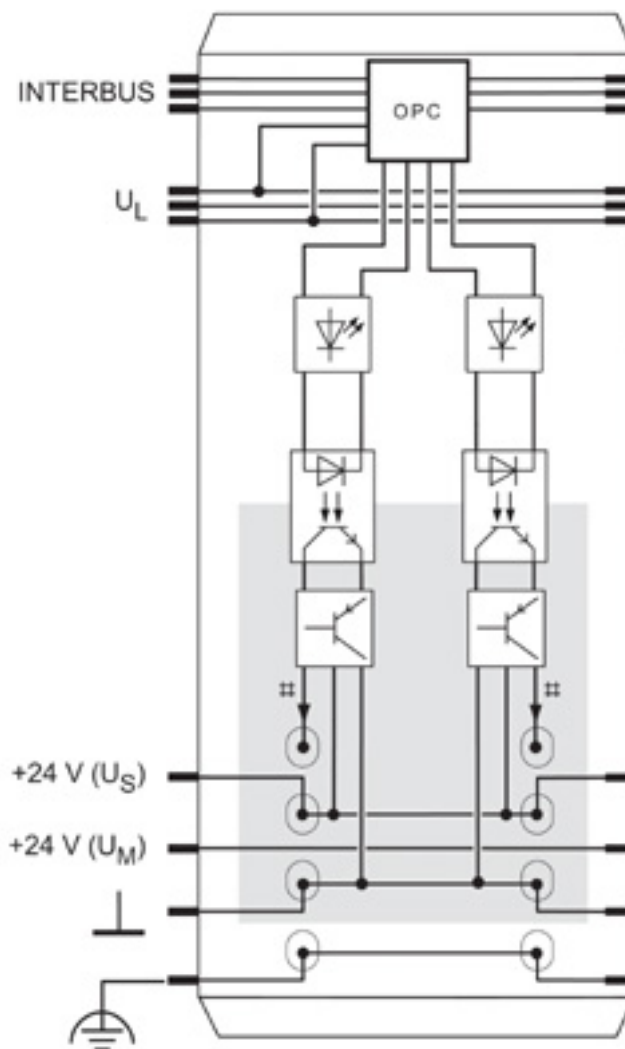
Schemat blokowy
