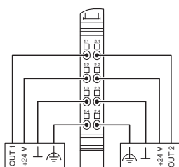
rysunek złączy
