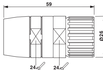
Rysunek wymiarowy
