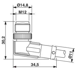
Rysunek wymiarowy
