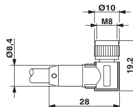
Rysunek wymiarowy
