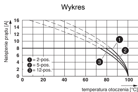
Typ: IMC 1,5/...-G-3,81 AU z MC 1,5/...-G-3,81 P... AU THR
