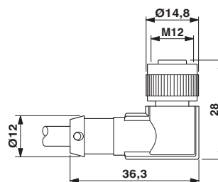
Rysunek wymiarowy
