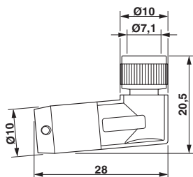
Rysunek wymiarowy
