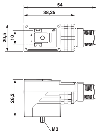
Rysunek wymiarowy
