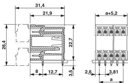
Rysunek wymiarowy
