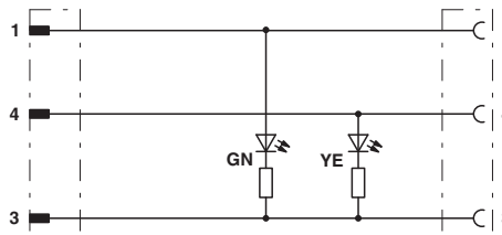
Przyporządkowanie styków wtyków / gniazd m8
