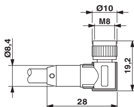
Rysunek wymiarowy
