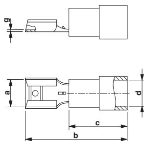
Rysunek wymiarowy
